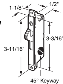
45° Keyway
