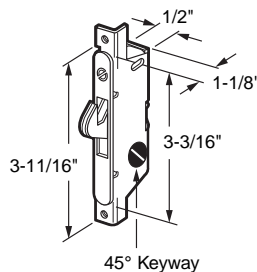
45° Keyway
